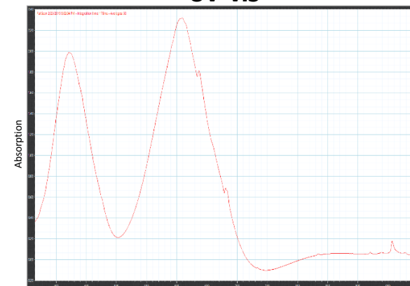
UV-vis
