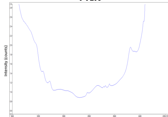
FTIR
