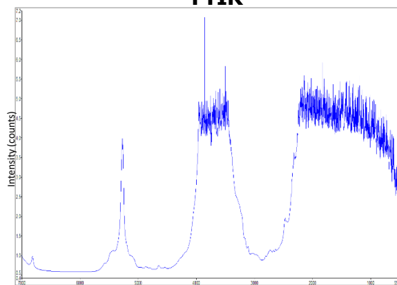
FTIR
